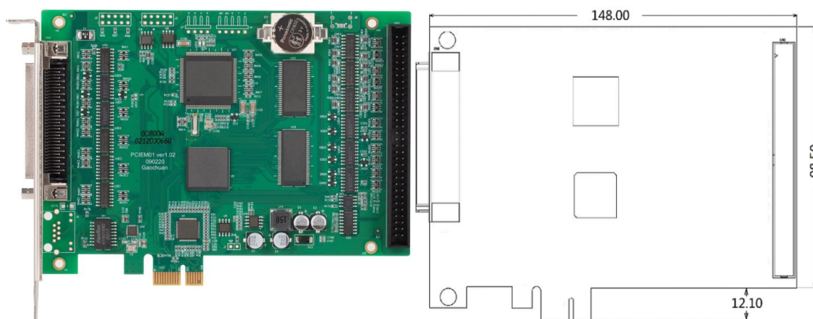
图 1.2.1 GCS160A-PCIE 控制卡主卡外观及尺寸图
