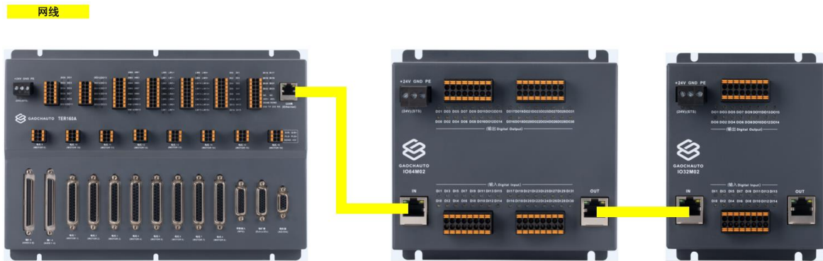
图 3.8.1 扩展模块接线示意图
