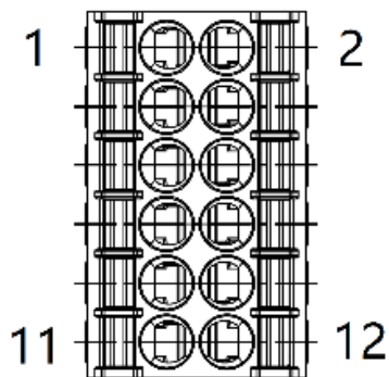
图 3.7.2 通用输出端子引脚顺序
