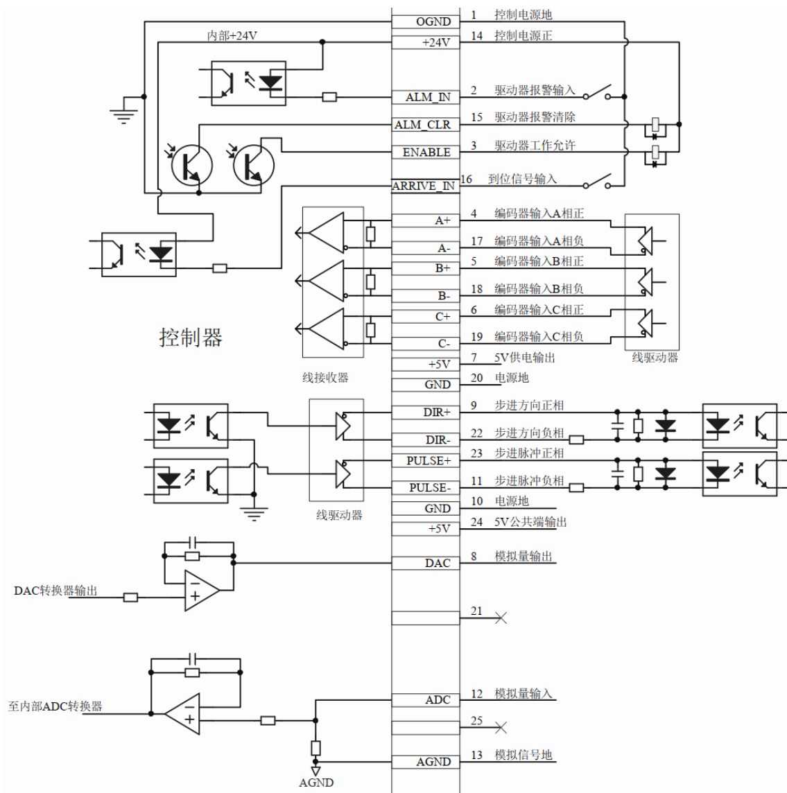
图 3.2.1 电机轴配线示意图
